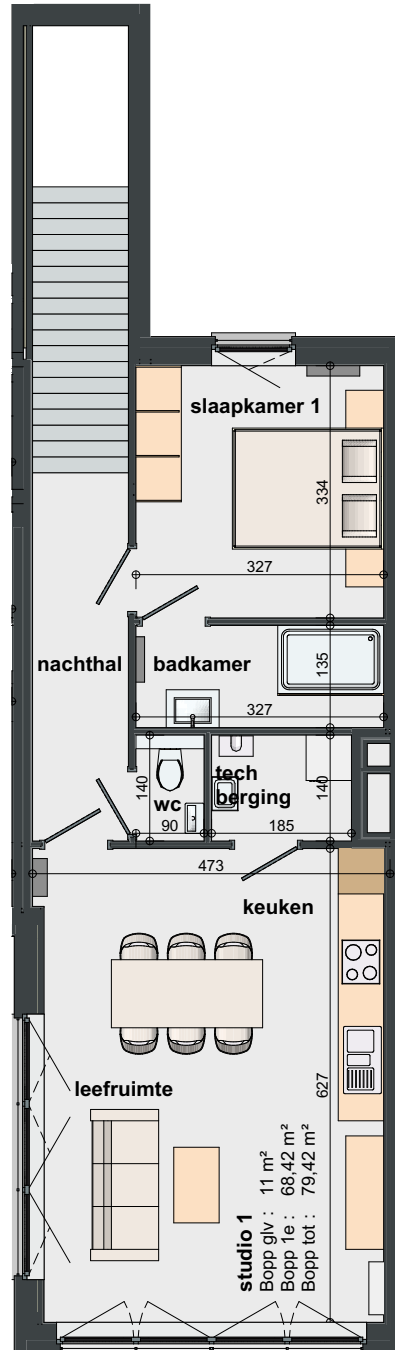
1e verdieping 1:100
