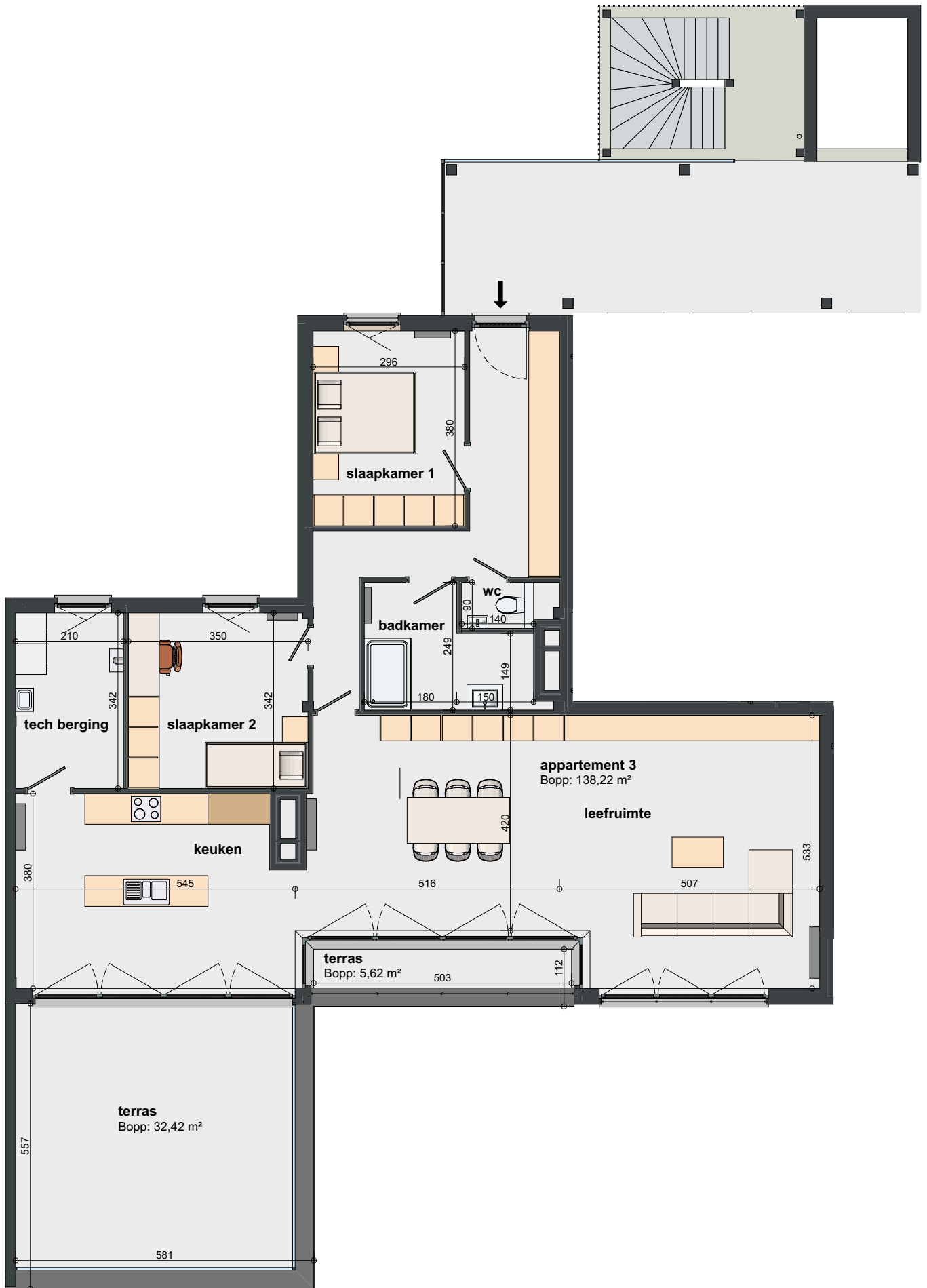
3e verdieping 1:100
